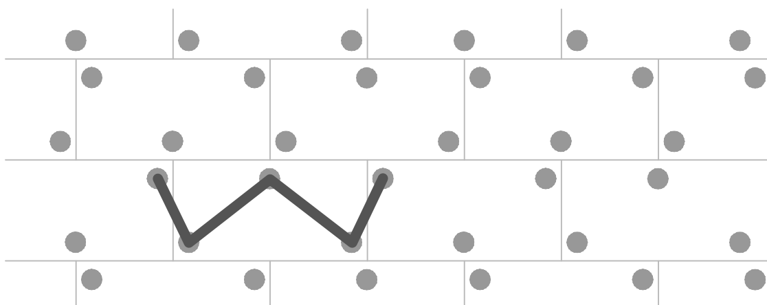
b) Esquema en W (paneles de lana mineral y lana de vidrio)
